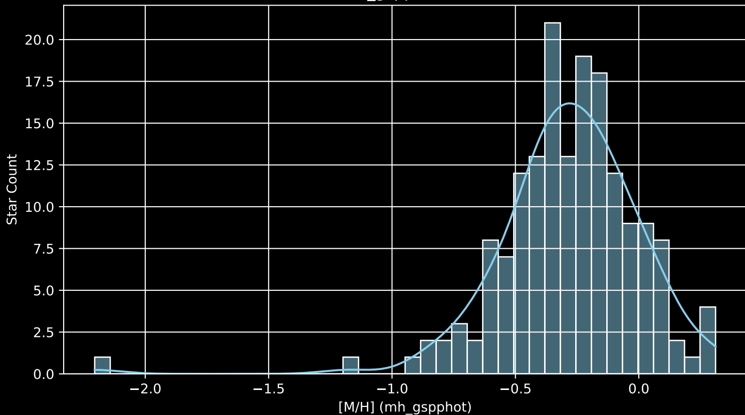
GALAH DR4 Field: [7126] [M/H] (mh_gspphot) (n= 168)
