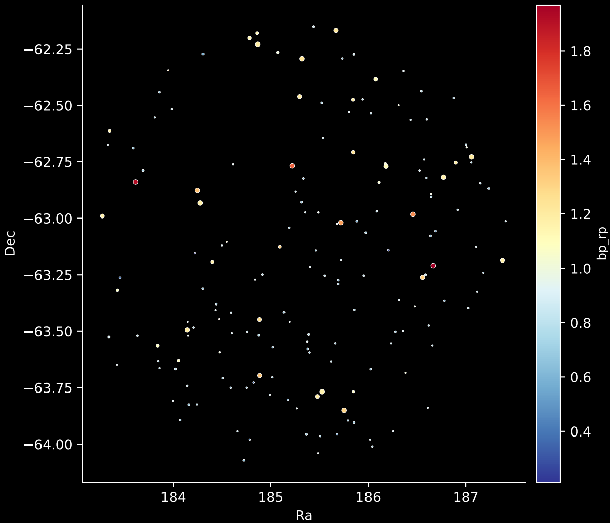
GALAH DR4 Field: [7126] Stars: 169
