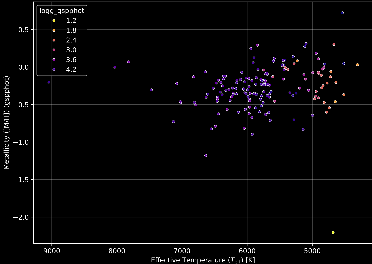
GALAH DR4 Field: [7126] Stellar Population Parameters (n= 169)
